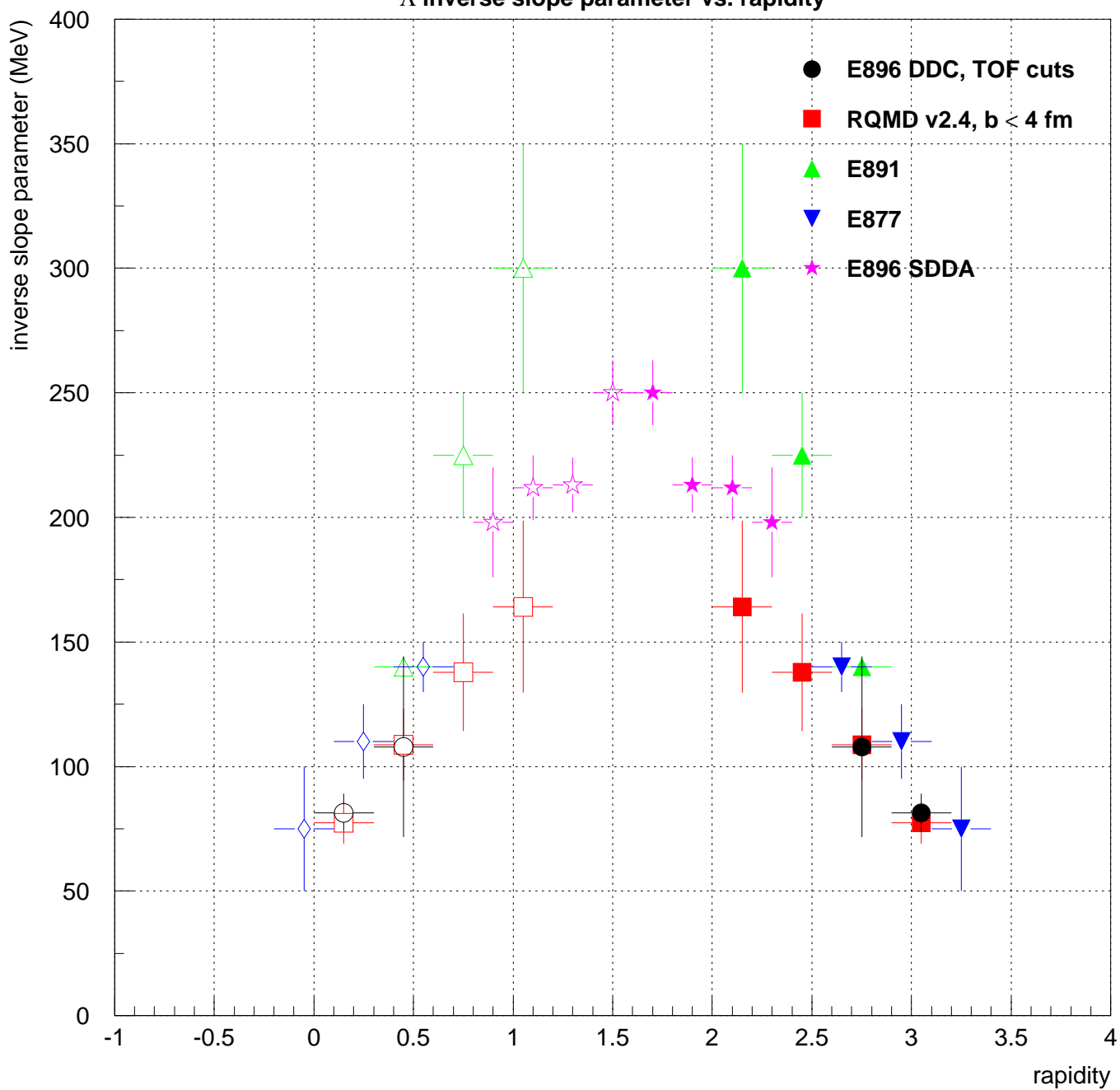
\Delta inverse slope parameter vs. rapidity
