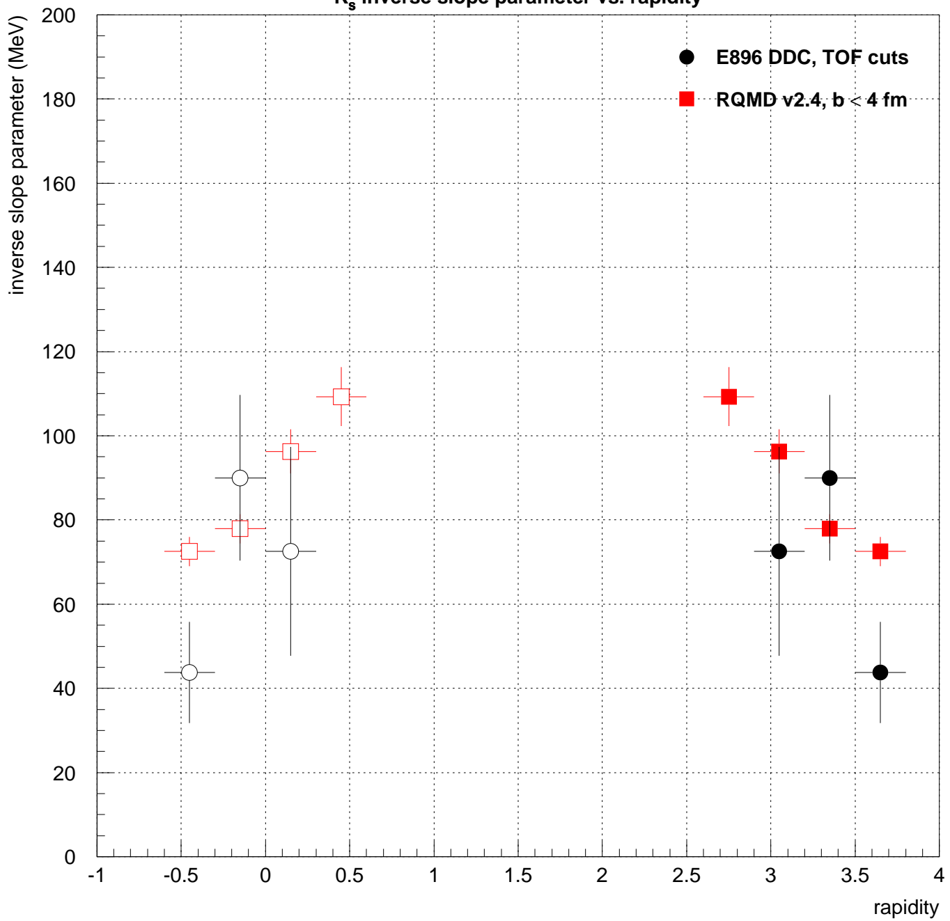
K_s inverse slope parameter vs. rapidity
