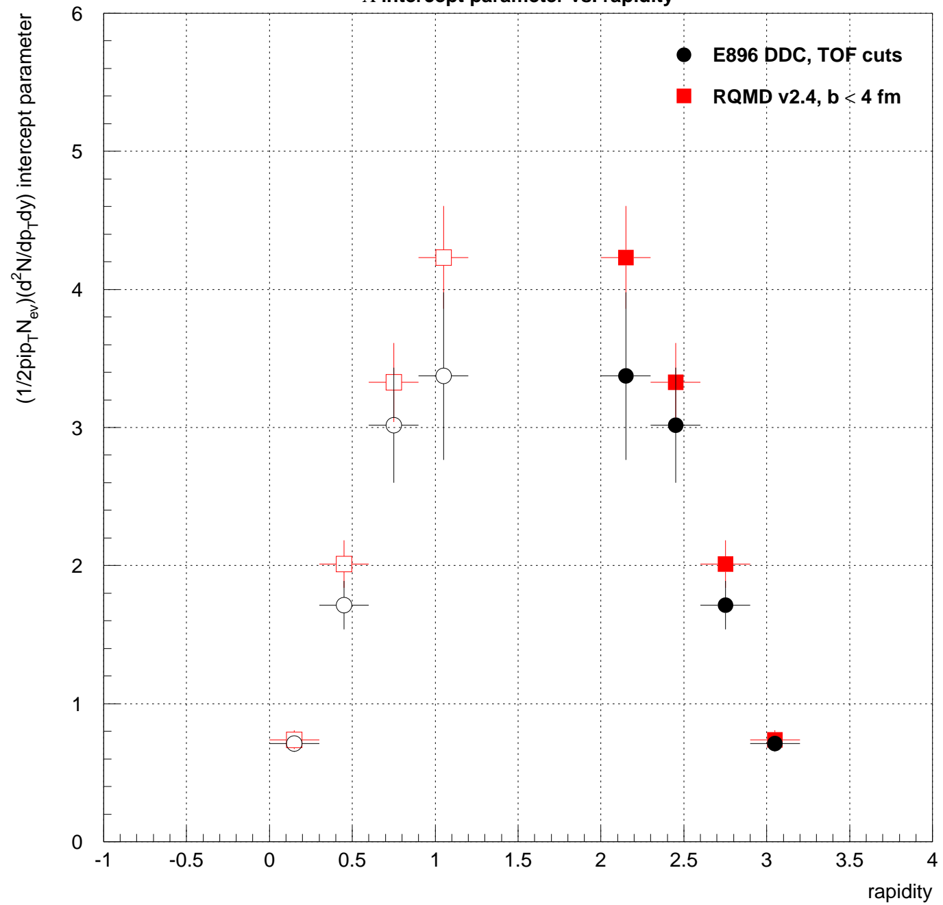
\Delta intercept parameter vs. rapidity
