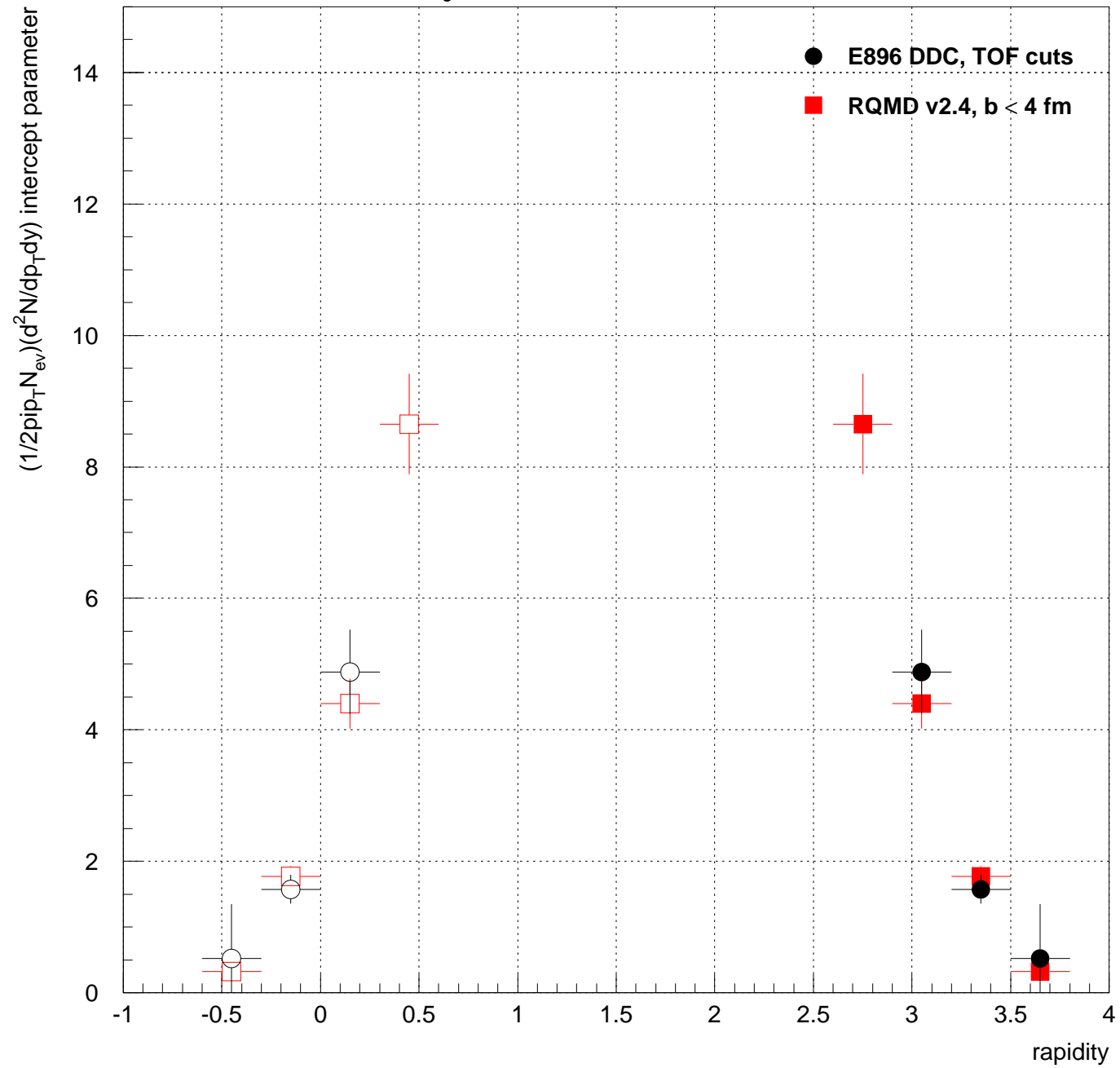
K_s intercept parameter vs. rapidity
